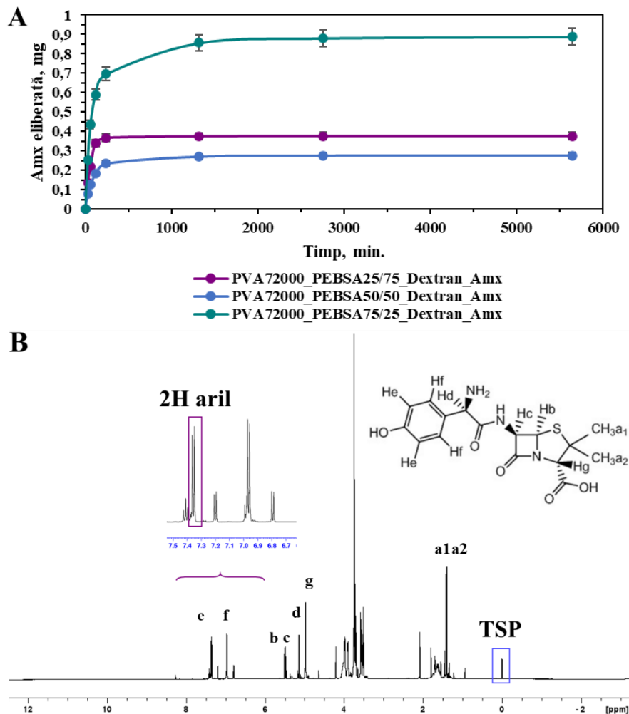
Figura 5.14. (A) Profilurile de eliberare ale Amx (mg) din hidrogelurile hibride pe bază de PVA 72000 _PEBSA_Dextran_Amx în soluții tampon fosfat salin pH = 7,4, de concentrație 0,01 M și (B) spectrul ^1\text{H} RMN @ 600 MHz sistemului PVA 72000 _PEBSA 25/75 _Dextran_Amx.
